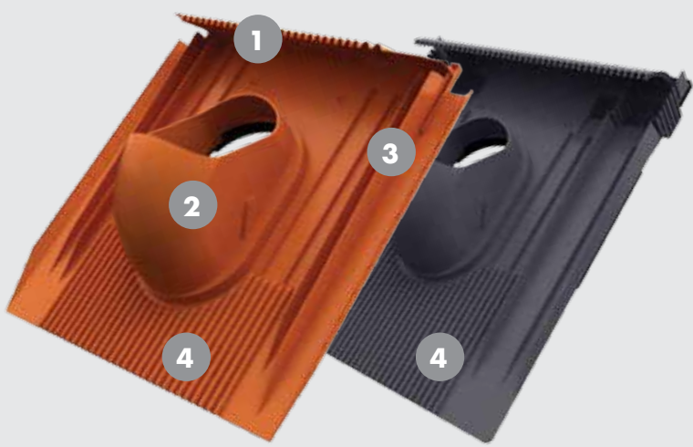
1 Regenkragen 2 Dom (für DN 110 oder DN 125) 3 Seitliche Paststreifen 4 Schürze (Standardausführung für flach bis mittel profilierte Dachziegel und Dachsteine, Decklänge 310 - 350 mm oder Ausführung mit längerer Schürze für stark profilierte Dachziegel und Dachsteine bis 60 mm, Decklänge 310 - 350 mm.
