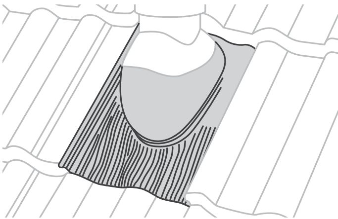
Universelle Grundplatte passt sich dank der flexiblen Schürze perfekt an das Profil der Dachpfanne an und wird links und rechts von den Dachpfannen eingedeckt.
